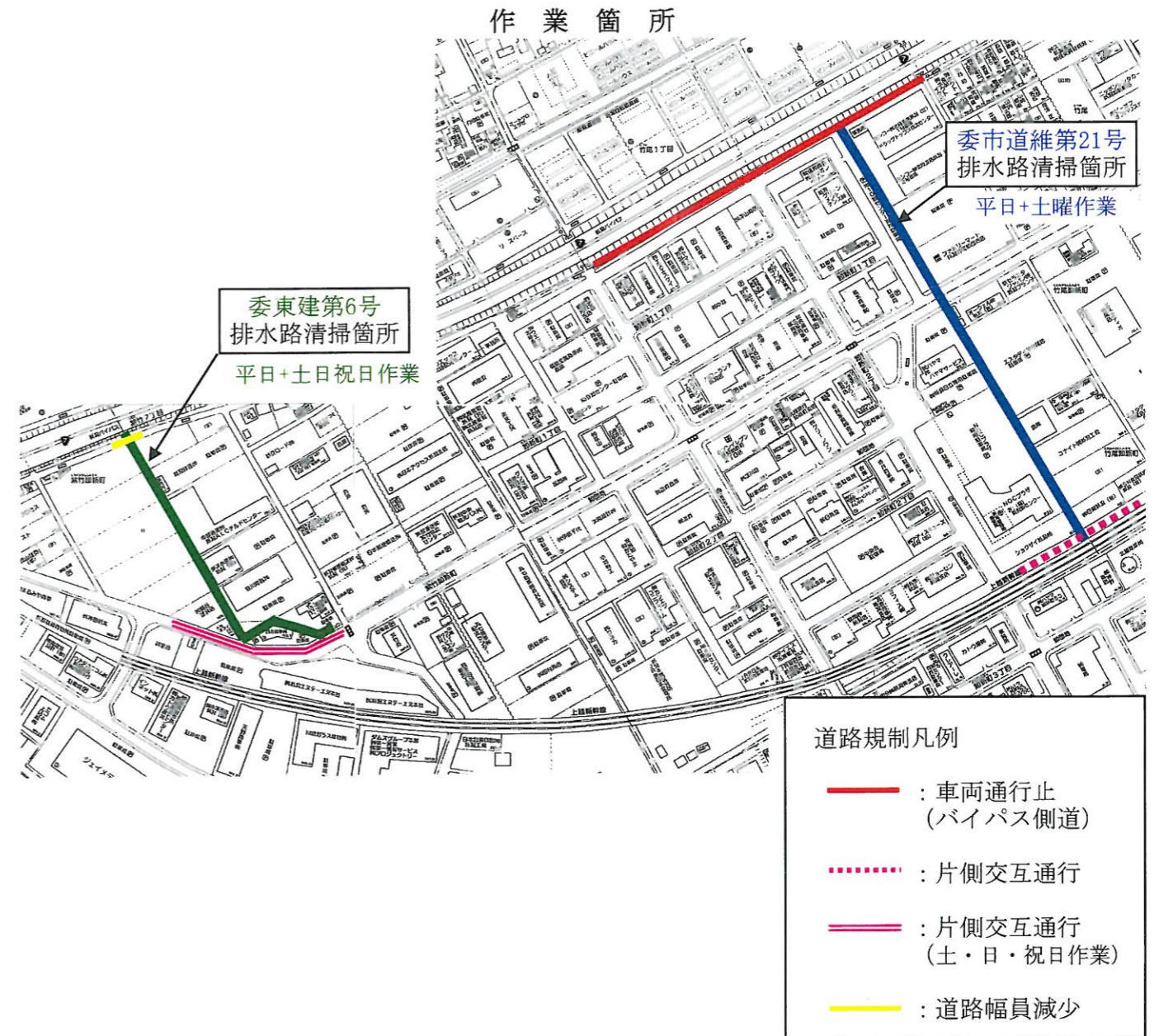
作業図
