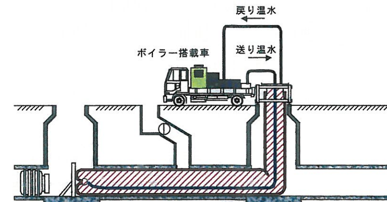
作業図
