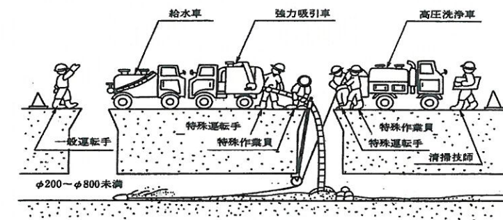
高圧洗浄車清掃作業標準図
