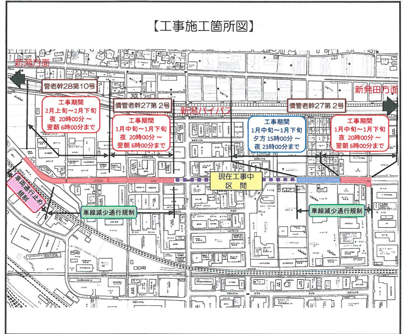
予定工程表 債管老幹27第2号 配水幹線布設工事 (株) ノガミ
