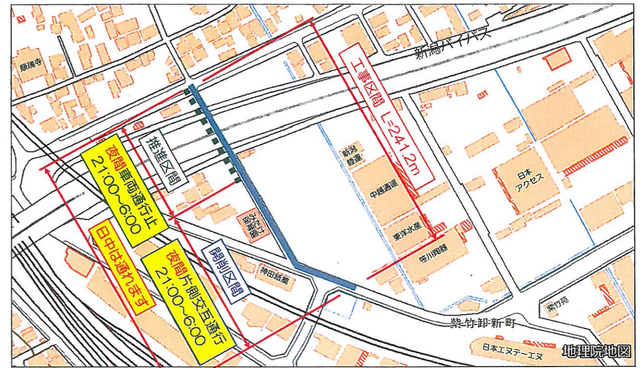
（ 工事箇所図 ）
