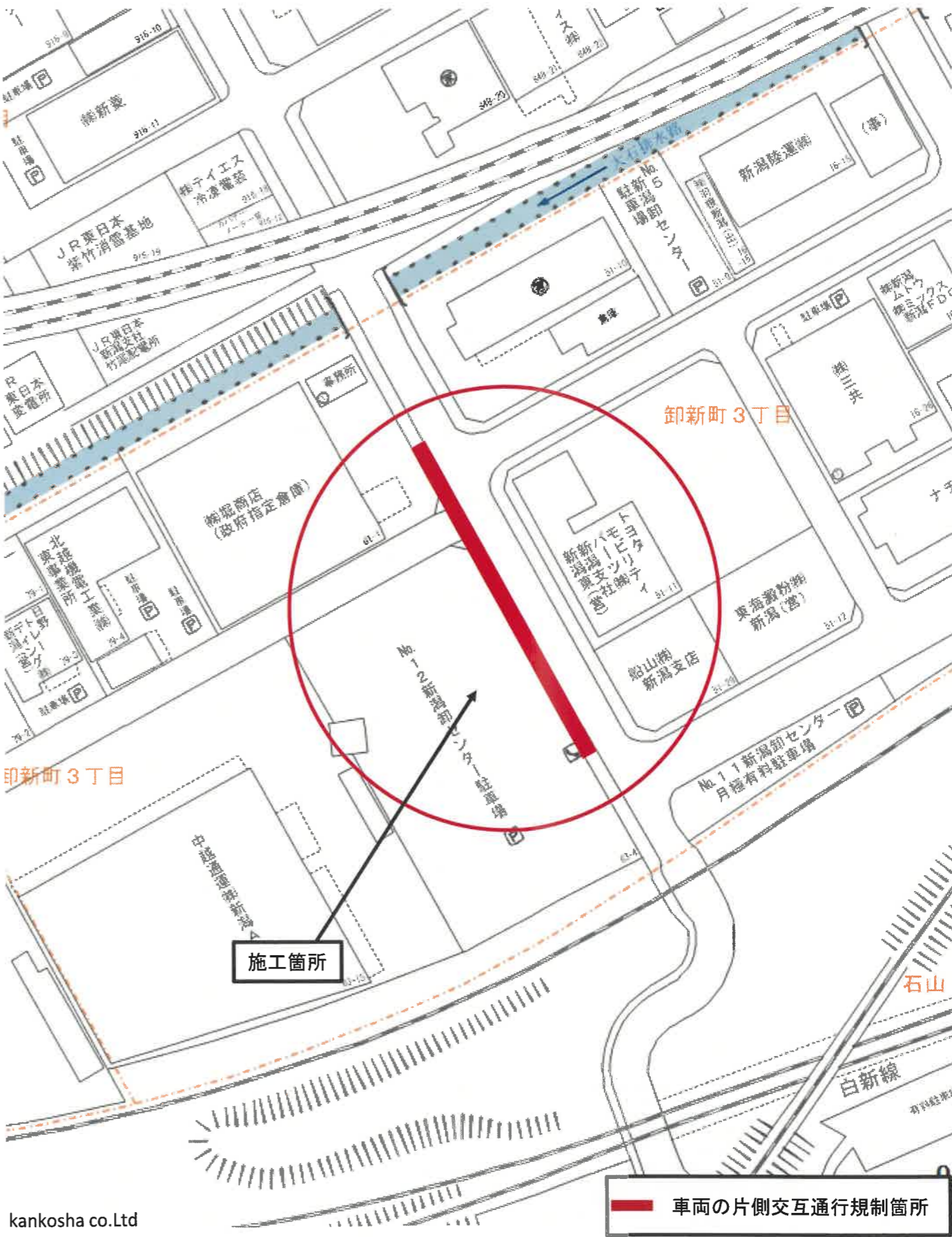
位置図
