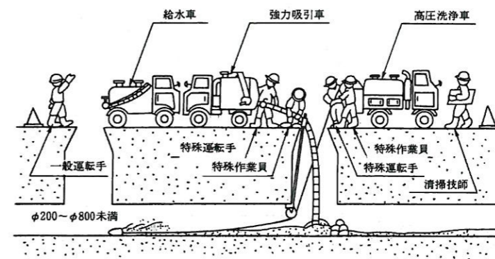
高圧洗浄車清掃作業標準図
